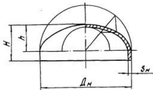
Заглушки из углеродистой стали
